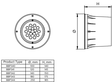
BBP340 LED220/WW 3W 20D 100-240V
