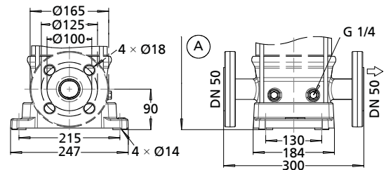
Movitec VF/VSF
