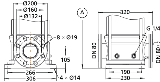
Movitec VF/VSF; PN 16, 25 - interchangeable range
