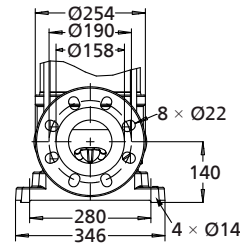
Movitec VF/VSF, PN 25/40
