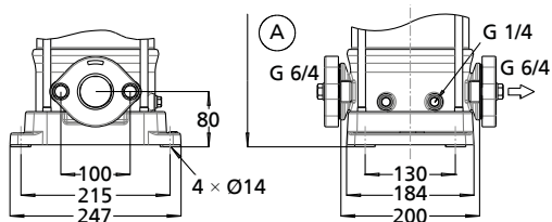
Movitec V/VS
