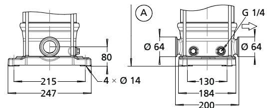
Movitec VT/VST
