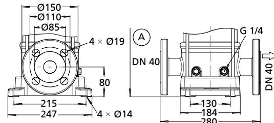
Movitec VF/SF
