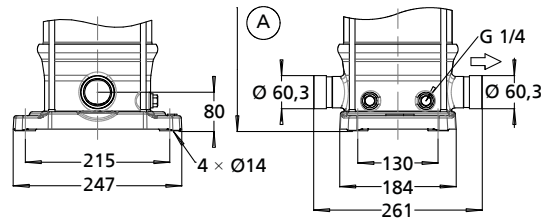
Movitec VV/SV
