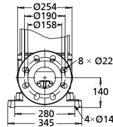
Movitec VCF, PN 25/40
